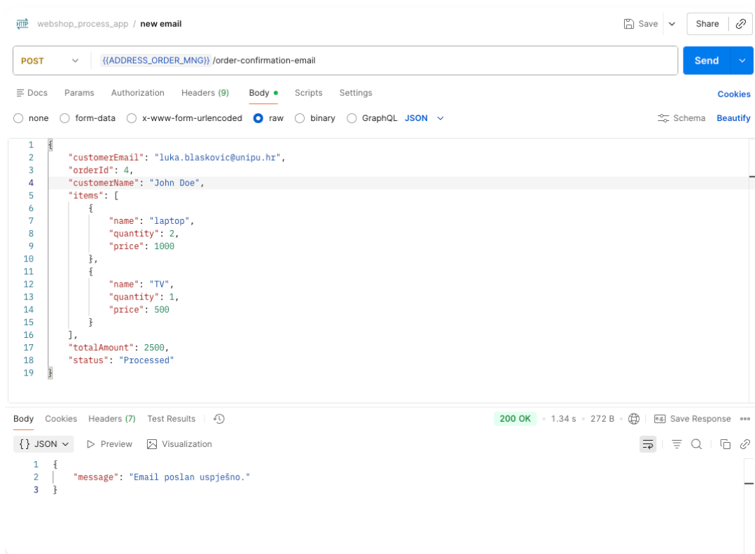
Slika 19. Testiranje slanja emaila putem Postmana koristeći novi endpoint POST /order-confirmation-email .
