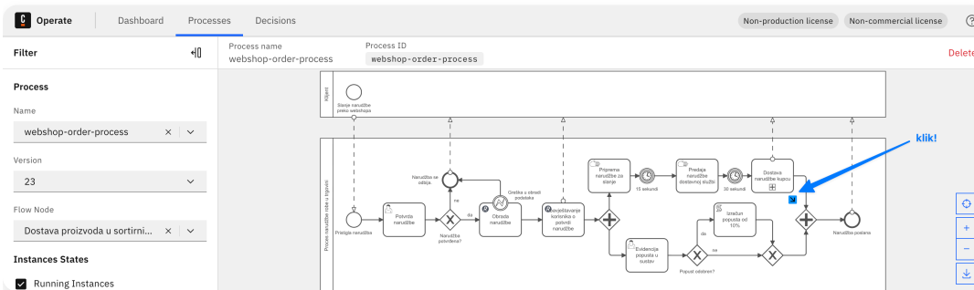
Slika 27. Pregled potprocesa unutar Camunda Operate aplikacije.
