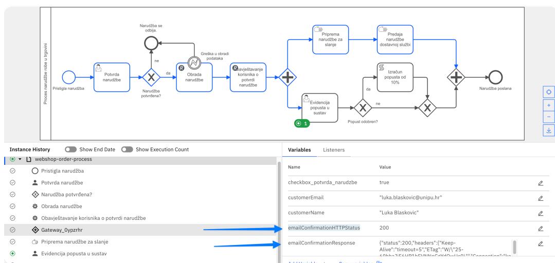
Slika 22. U Camunda Operate aplikaciji možemo vidjeti da je otpremni zadatak "Obavještanje korisnika o potvrdi narudžbe" uspješno izvršen.
