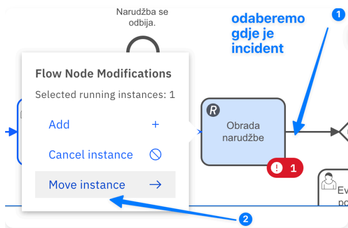
Slika 10. Unutar Camunda Operate aplikacije odaberite Modify Instance, a potom Move instance da biste preusmjerili tok procesa na drugu aktivnost.
