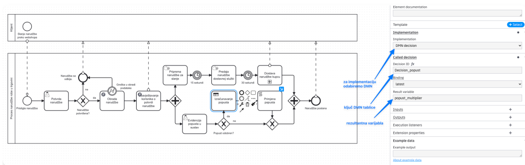
Slika 30. Dodavanje Business Rule Taska za povezivanje s DMN tablicom odluka.
